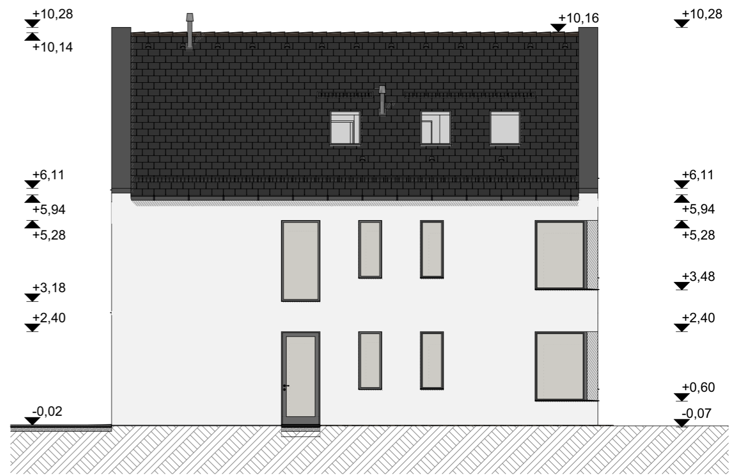
NY homlokzat 1:100
