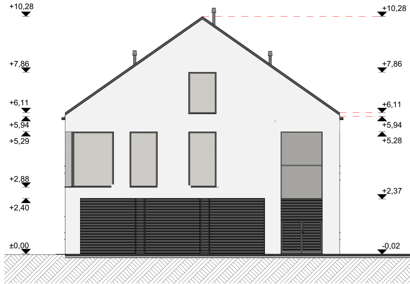
É homlokzat 1:100
